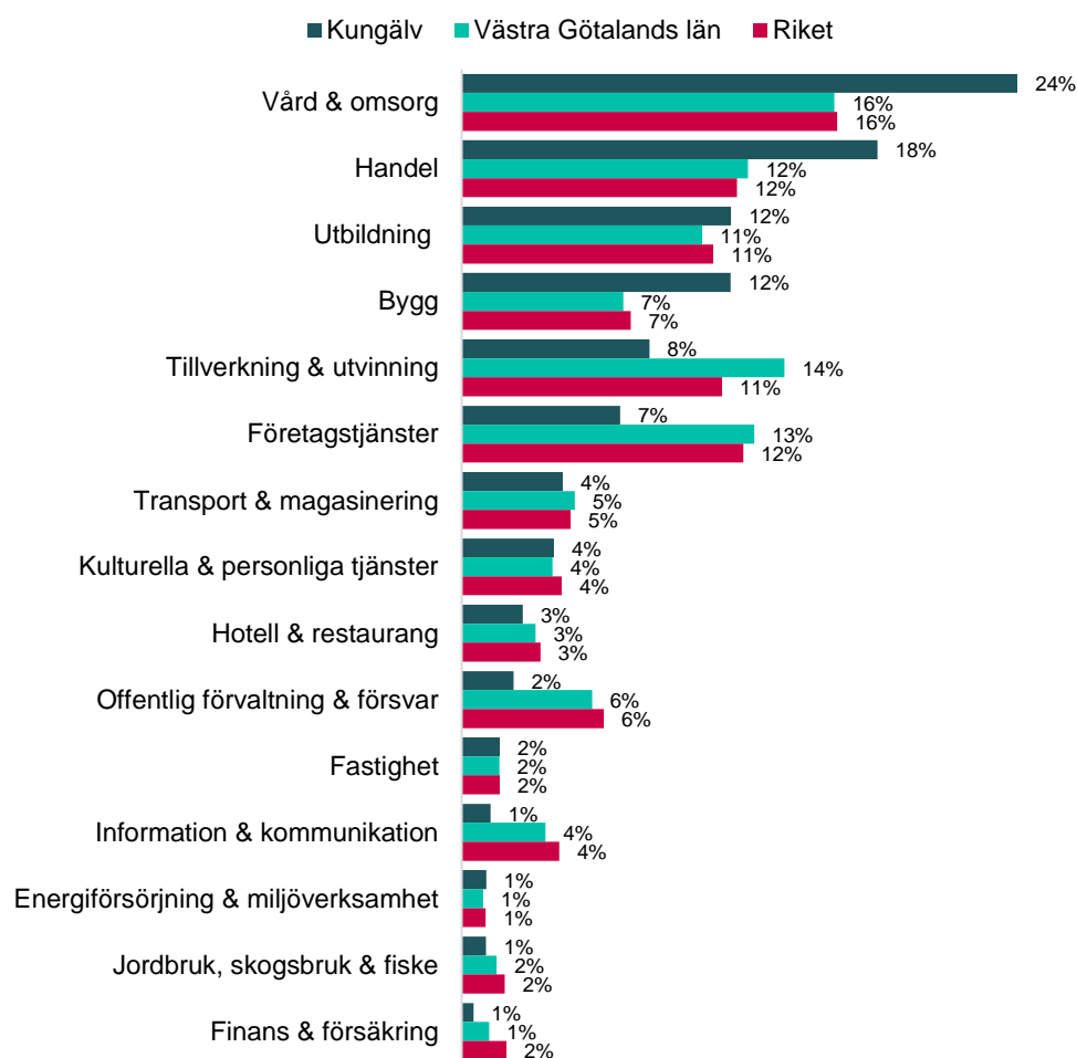
Figur 21 - Sysselsatta per bransch i Kungälv kommun, 2018
