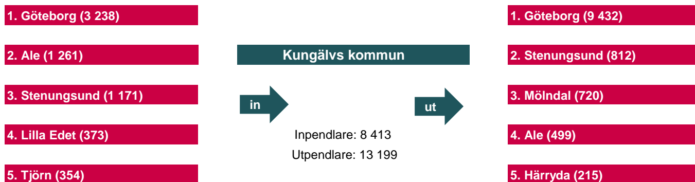
Figur 16 - Pendling från och till Kungälv kommun
